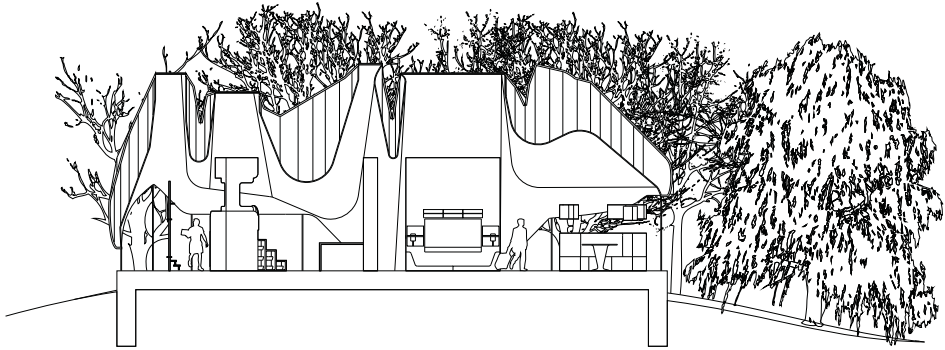
Longitudinal Section
